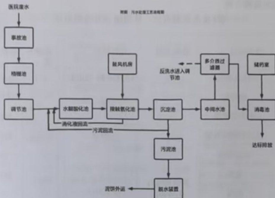
附图：污水处理站工艺流程图
